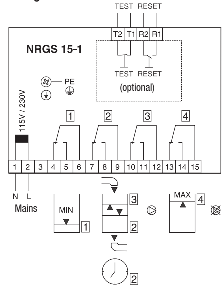
Fig. 2 Wiring diagram
